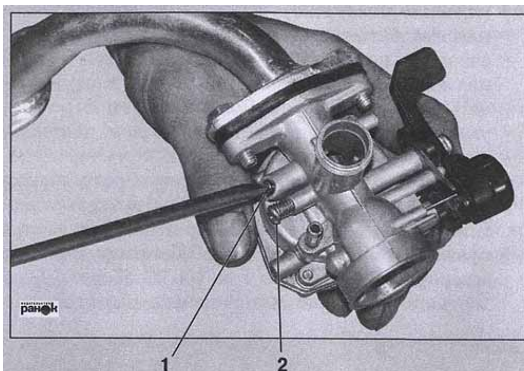
Рис. 29. Регулировка оборотов холостого хода карбюратора (для удобства показано на снятом карбюраторе): 1 – винт регулировки состава смеси (винт качества); 2 – винт регулировки частоты вращения коленчатого вала на холостом ходу (винт количества)
