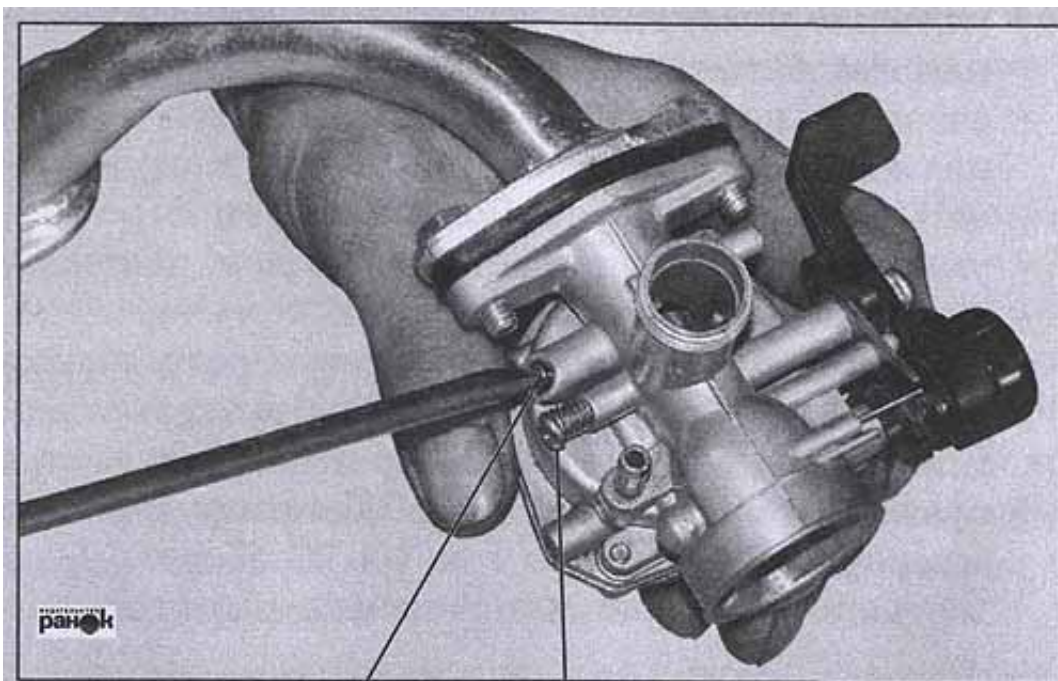
Рис. 29. Регулировка оборотов холостого хода карбюратора (для удобства показано на снятом карбюраторе): 1 – винт регулировки состава смеси (винт качества); 2 – винт регулировки частоты вращения коленчатого вала на холостом ходу (винт количества)
